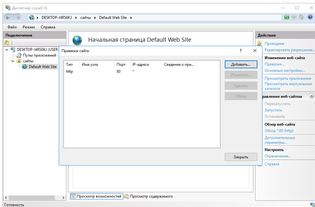
Рисунок 106. Привязки сайта
