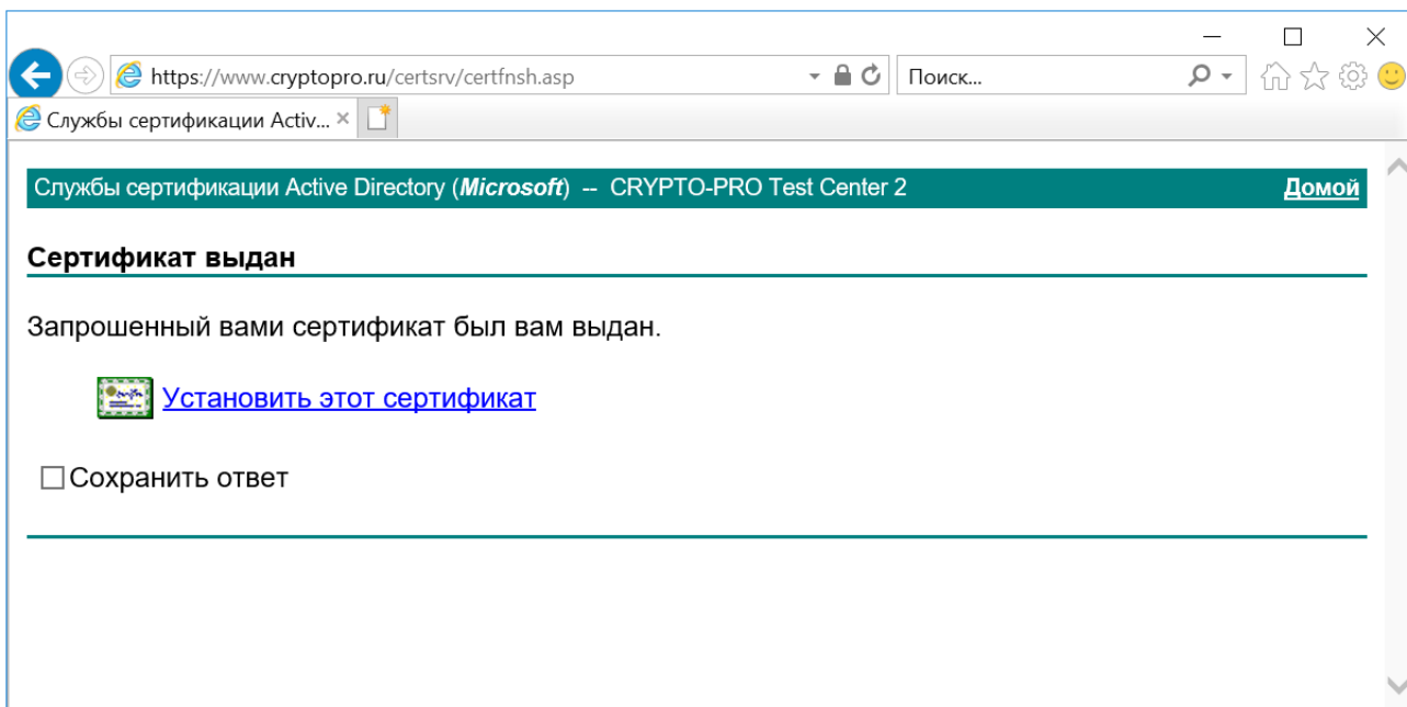
Рисунок 90. Установка сертификата
