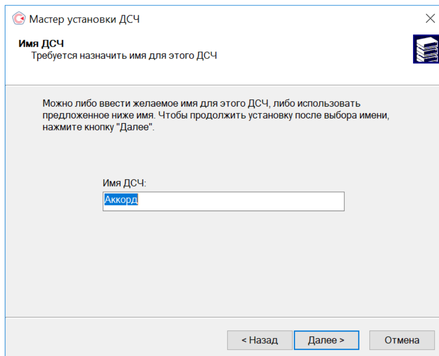
Рисунок 42. Имя ДСЧ
