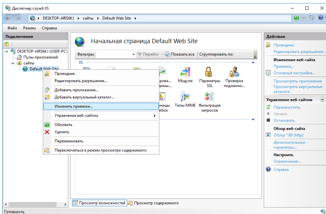
Рисунок 105. Диспетчер IIS
