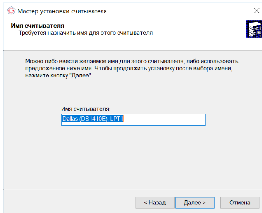
Рисунок 25. Имя считывателя
