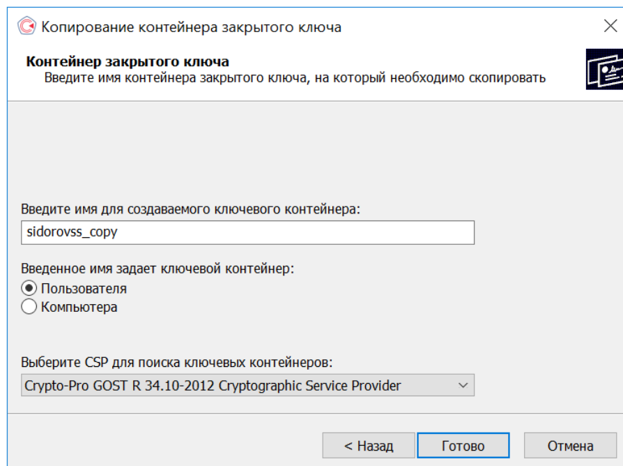
Рисунок 53. Ввод имени нового контейнера
