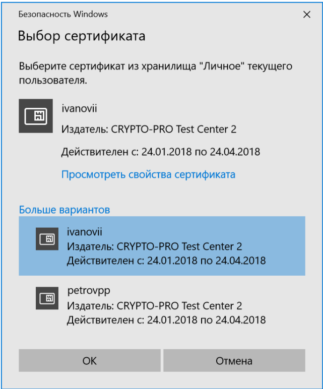
Рисунок 50. Выбор сертификата
