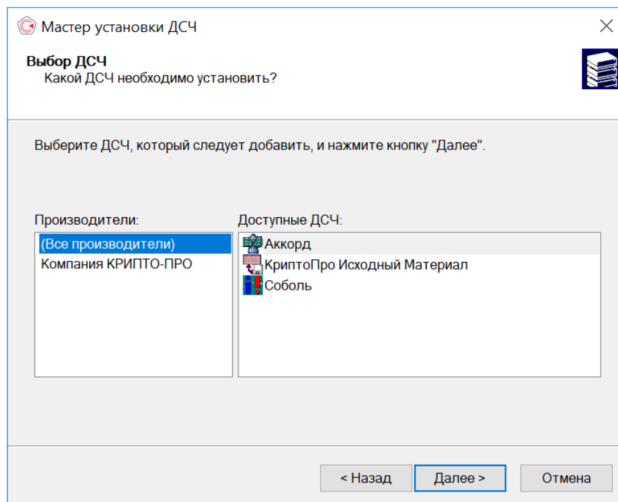
Рисунок 41. Выбор ДСЧ
