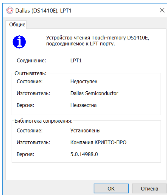
Рисунок 29. Свойства считывателя
